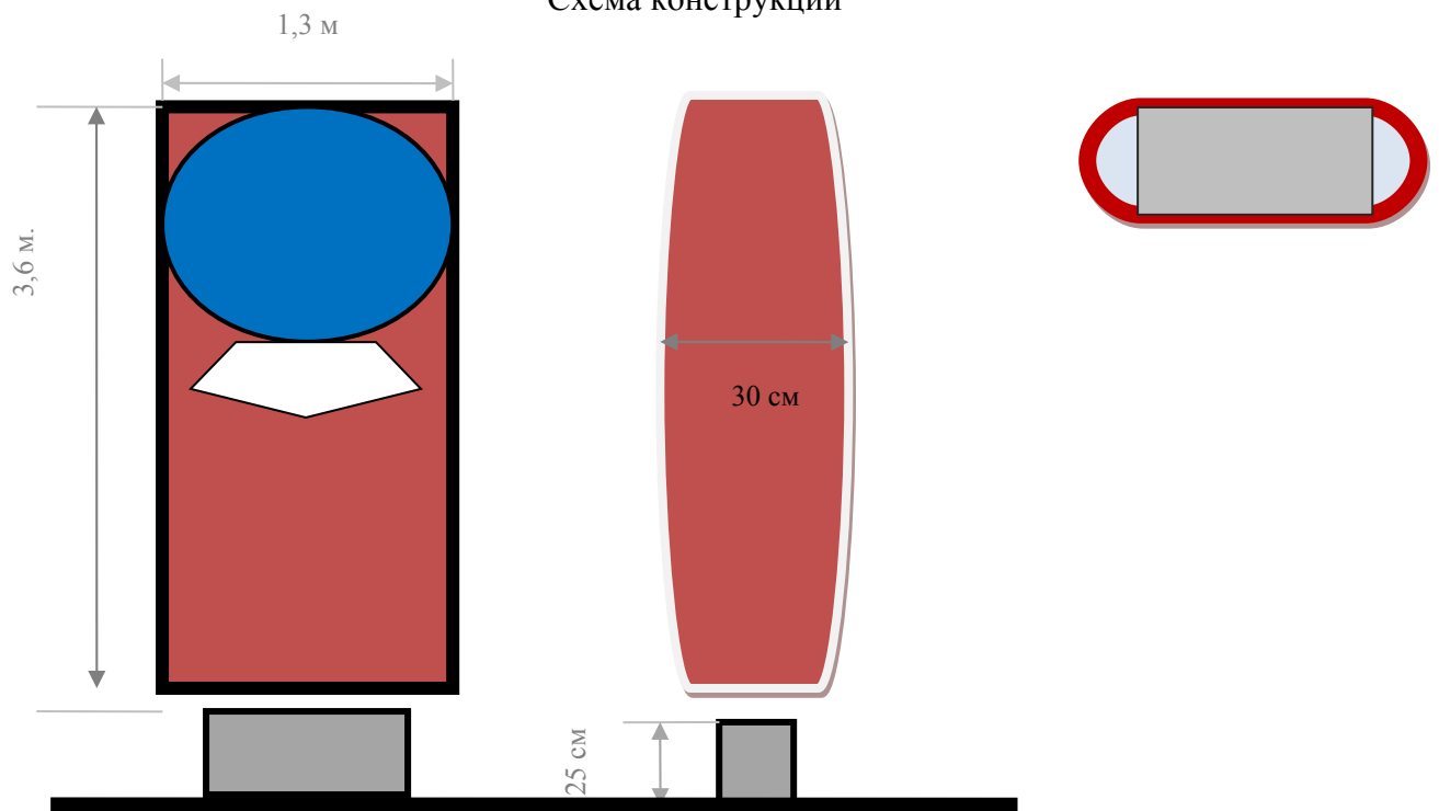
Схема конструкции
