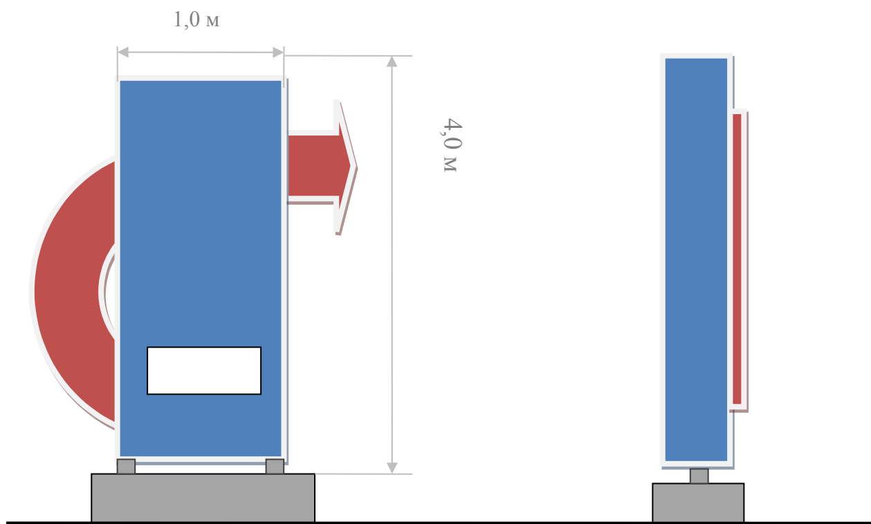
Схема конструкции
